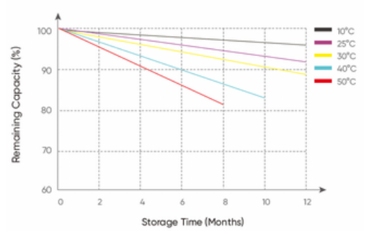
Farklı Sıcaklıklara Göre Kendiliğinden Deşarj Eğrisi
