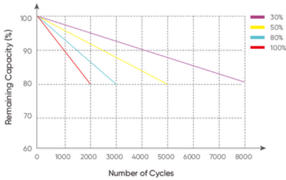
Farklı DOD Deşarj Döngüsü Ömür Eğrisi (0,5C)
