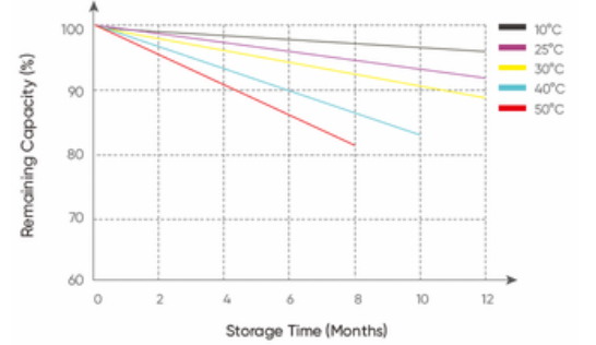
Farklı Sıcaklıklara Göre Kendiliğinden Deşarj Eğrisi
